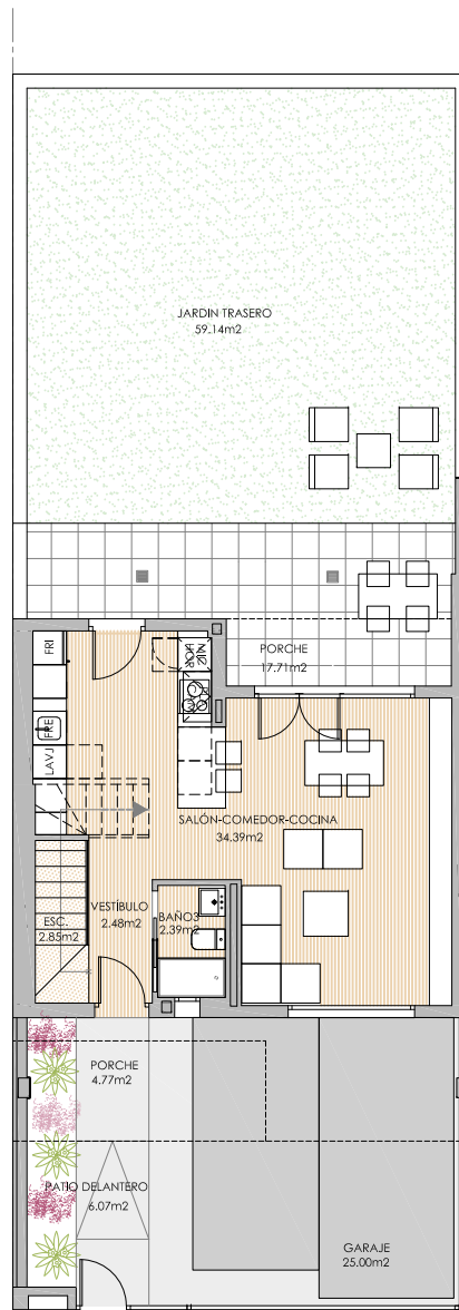
PLANTA BAJA
