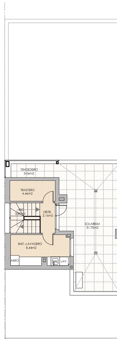
PLANTA CUBIERTA
